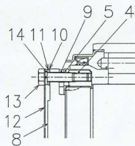
ア部詳細 (R 1/2 )
