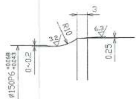
工部詳細 (尺度 \frac{1}{1} )
