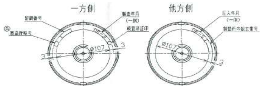
ア部詳細 (尺度 \frac{1}{2} )
