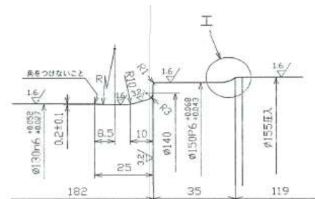
ウ部詳細 (尺度 \frac{1}{1} )
