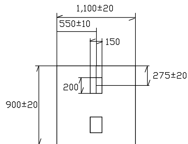
上面図
