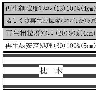
〔交差点部構造図(37kgレール区間)〕
