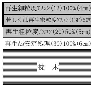
〔交差点部構造図(50Nレール区間)〕
