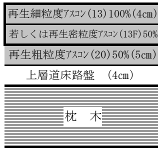
〔一般部構造図(37kgレール区間)〕
