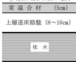
〔欠損部補修断面(1層)〕
