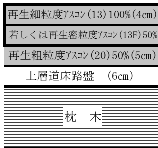
〔一般部構造図(50Nレール区間)〕
